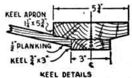
KEEL DETAILS
